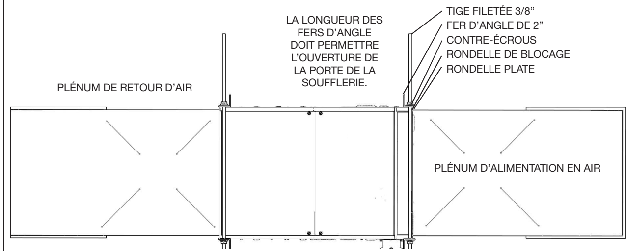
FIGURE 3 - MÉTHODE SUGGÉRÉE DE SUSPENDRE LA FOURNAISE HORIZONTALE
