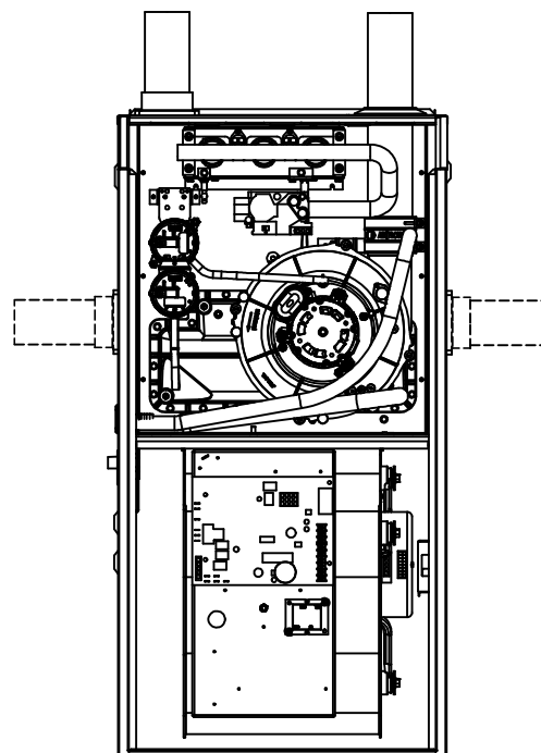
FIGURE 16 - OPTION D'ÉVACUATION ET DE COURANTE ASCENDANTE
