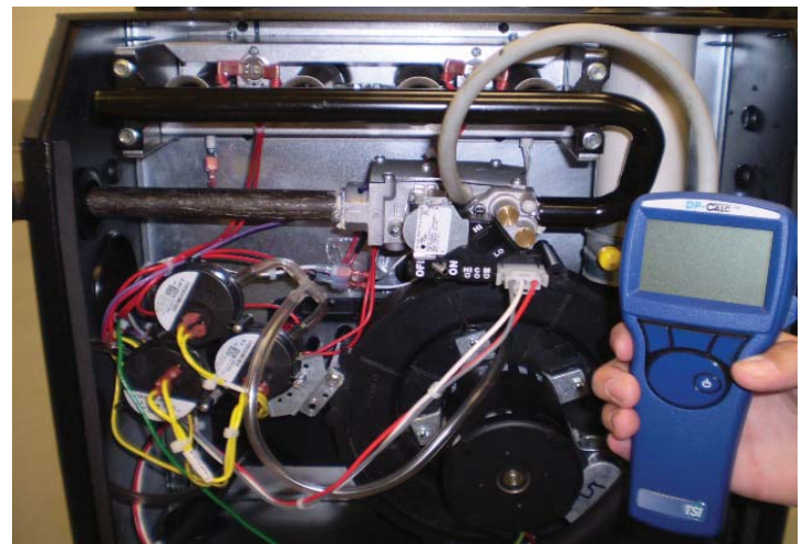
FIGURE30 - MANOMÈTRE QUI MESURE LA PRESSION DU GAZ AU COLLECTEUR
