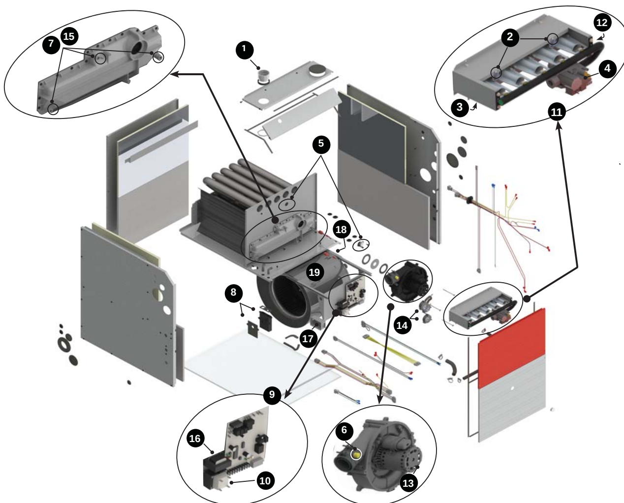
FIGURE 2 - COMPOSANTS DE LA FOURNAISE
