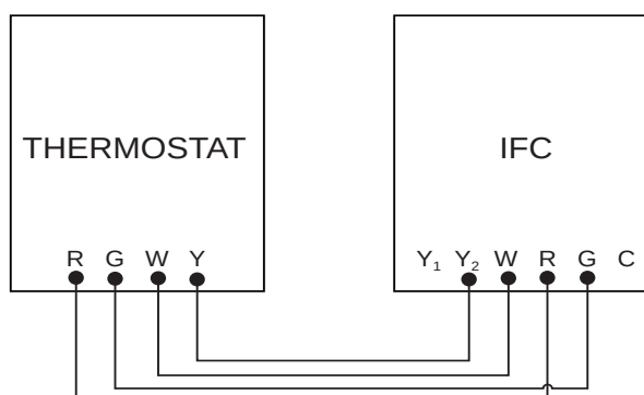
FIGURE 33 - DIAGRAMME DU CONNECTION DU THERMOSTAT
