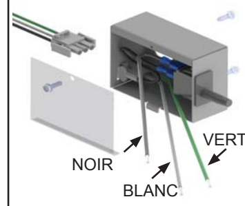
FIGURE 31 - BRANCHEMENTS ÉLECTRIQUES/CONNECTEUR MOLEX
