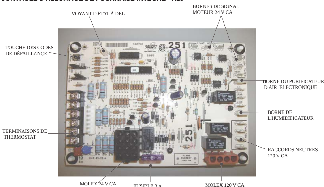
FIGURE 32 - CONTRÔLE D'ALLUMAGE DE FOURNAISE INTÉGRÉ - X13
