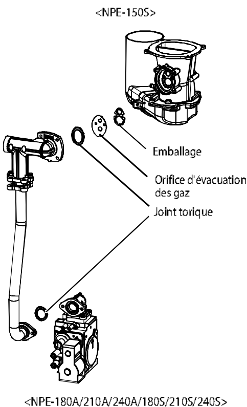
Figure 5. Vue éclatée du tuyau à gaz
