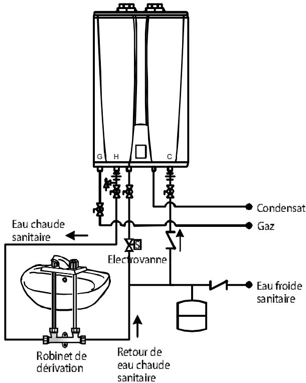
Mode de recirculation externe utilisant un robinet de dérivation
