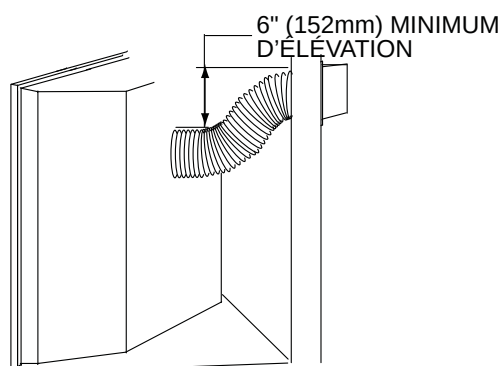
Évent Flexible
