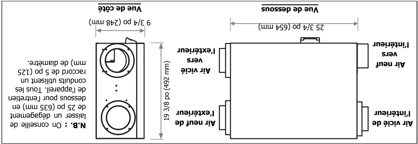
Dessin dimensionnel pour le modèle AIR125ERV
